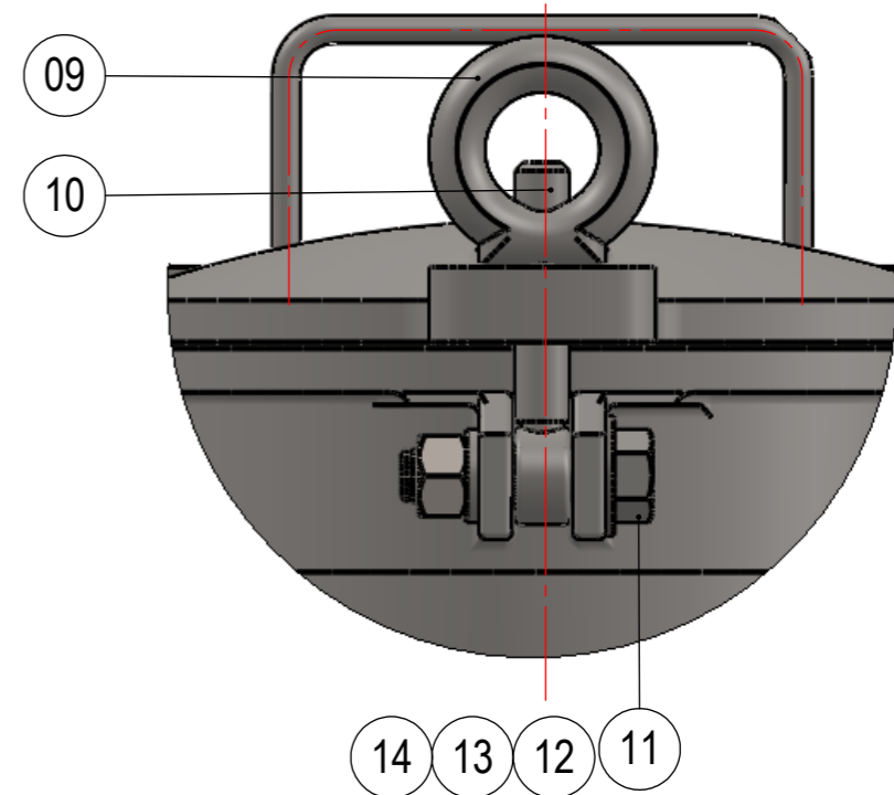
DETALHE D ESCALA: 1 : 2
