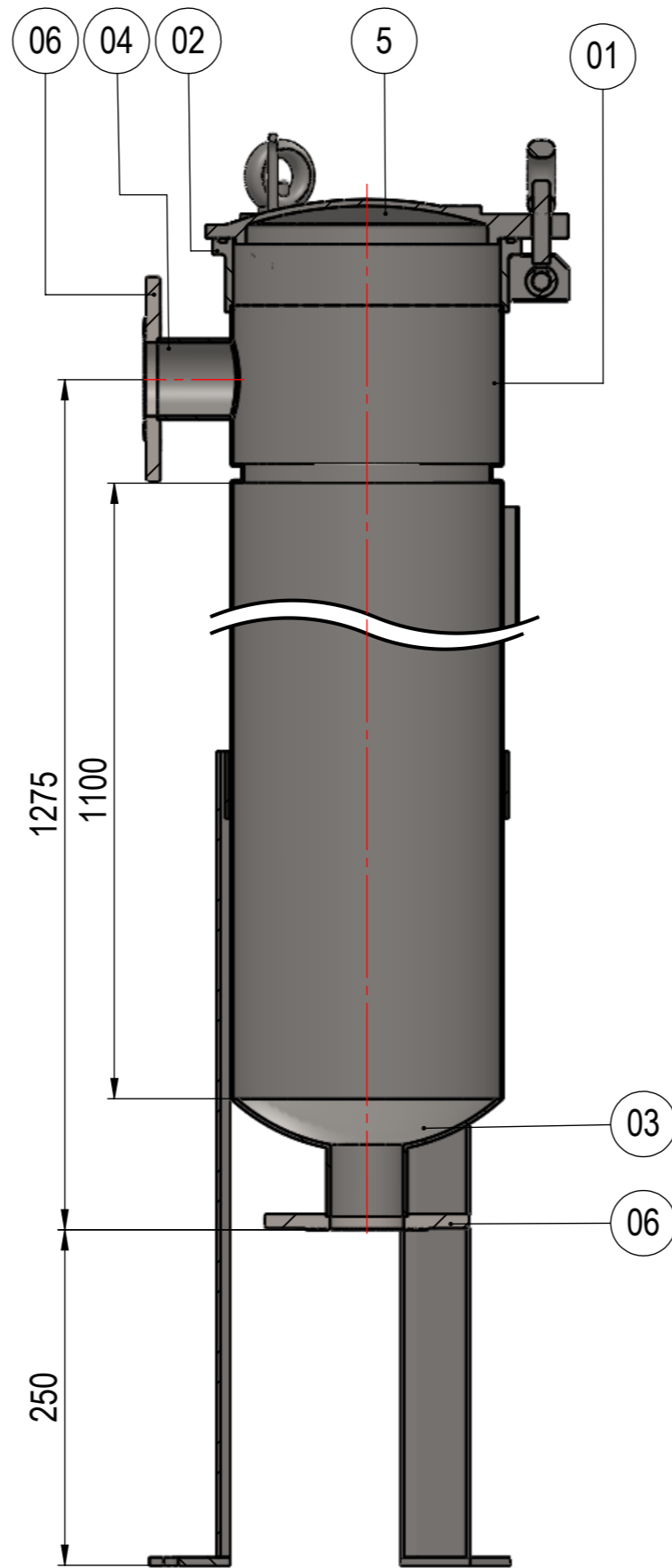
CORTE A-A
