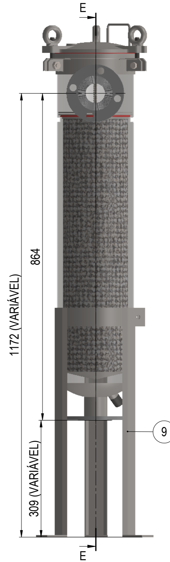
DETALHE C ESCALA: 1 : 3
